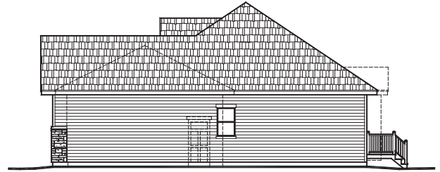
RIGHT ELEVATION
