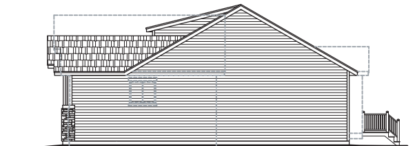
RIGHT ELEVATION
